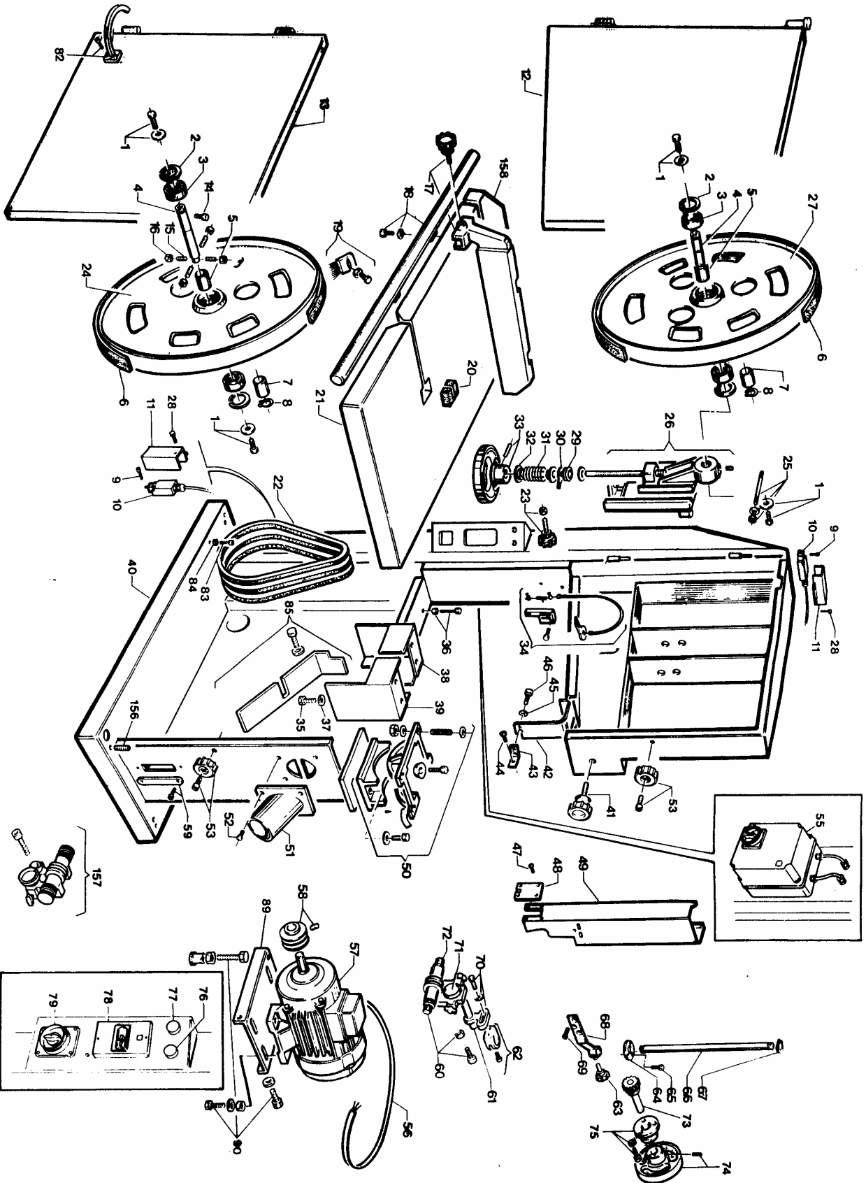
PEZZI DI RICAMBIO MODELLI SR-DS 800/900 CE
